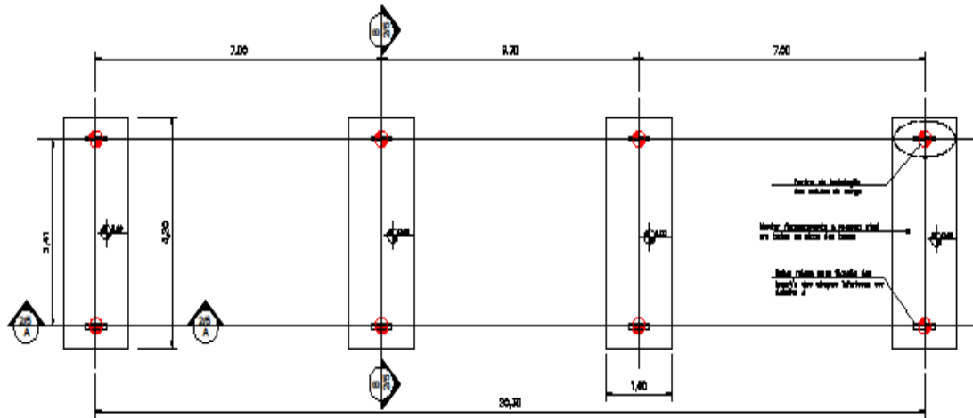
PLANTA BAIXA
